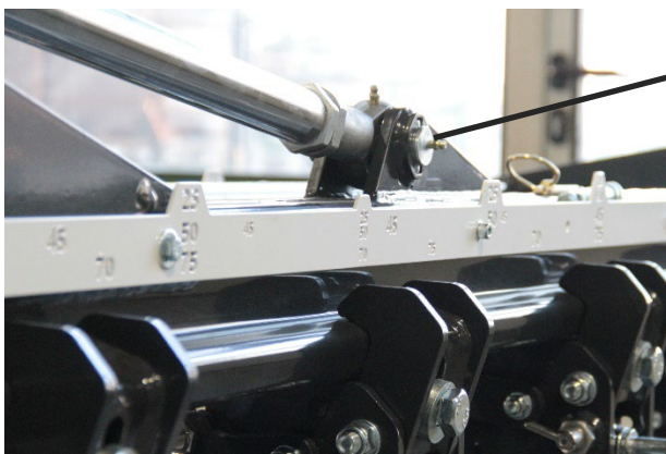
Abbildung 41: Klappzylinder
