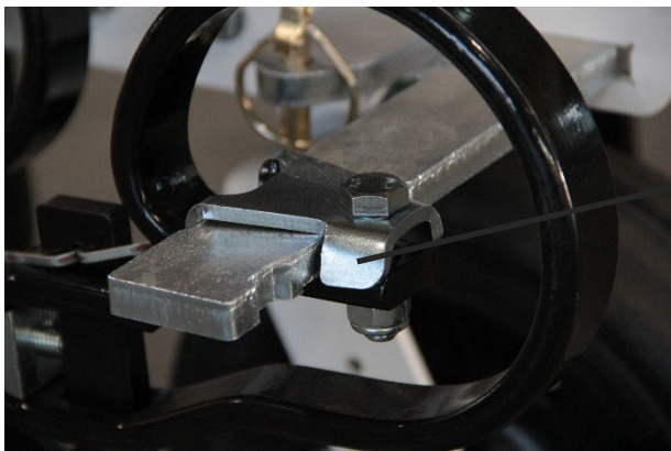
Abbildung 20: Federzinkenklemmung
