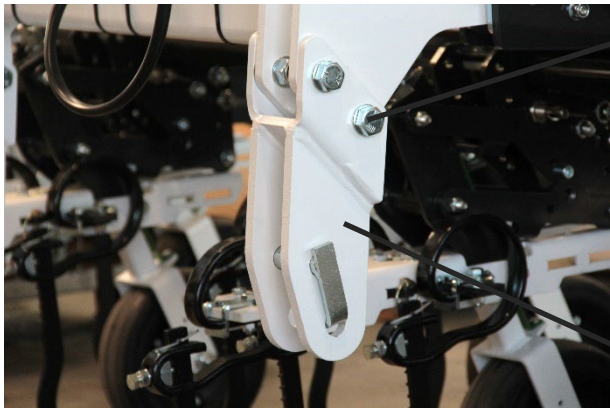
Abbildung 5: Unterlenkeranhangung
