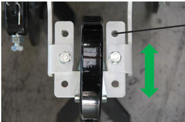
Abbildung 18: mittiger Zinken
