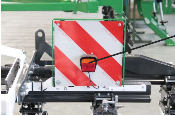
Abbildung 36: Heckbeleuchtung
