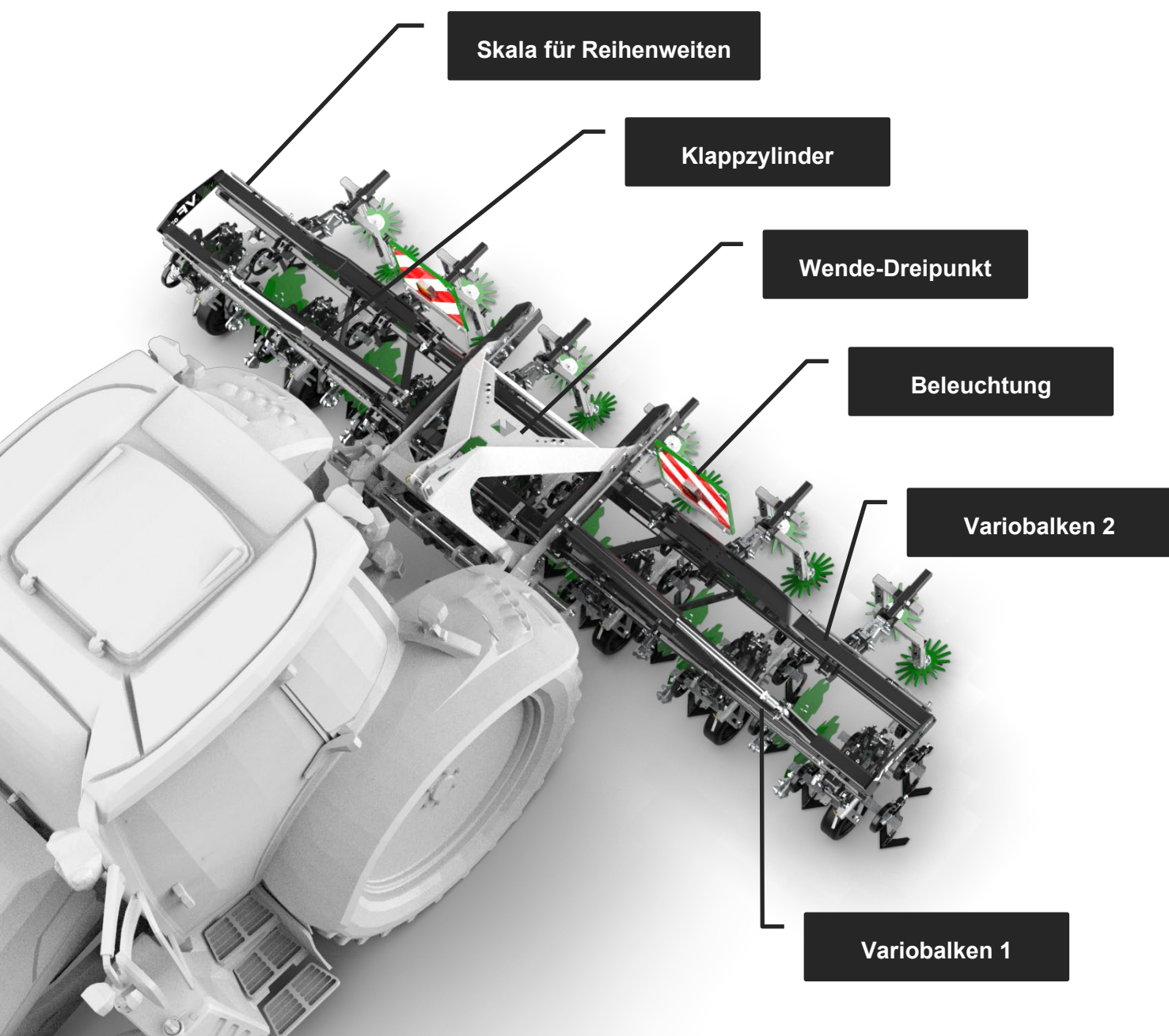
Abbildung 1: Aufbau Variofield
