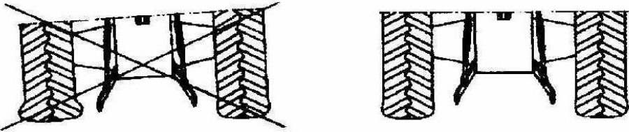
Abbildung 38: Reifenluftdruck
