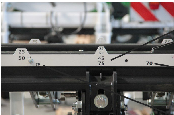
Abbildung 6: Reihenweitenskala
