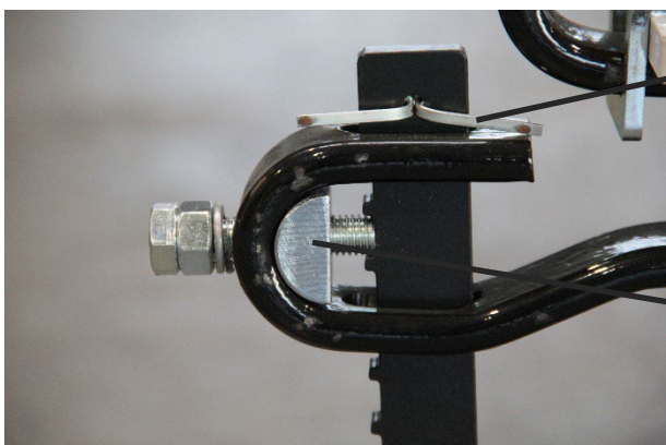
Abbildung 19: Stielklemmung
