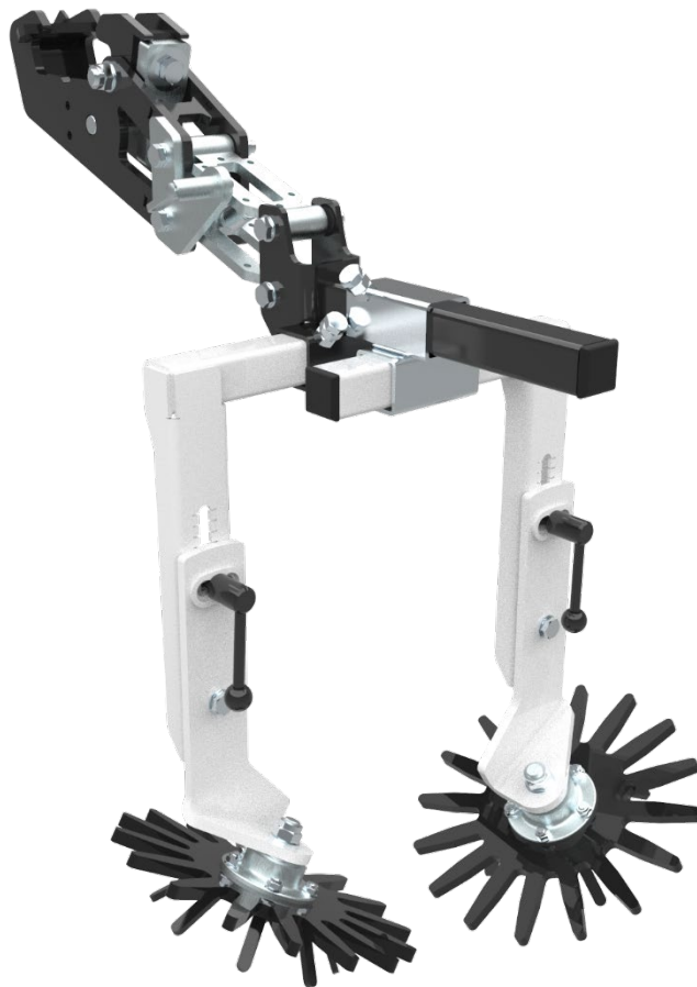
Abbildung 29: Fingerhackmodule
