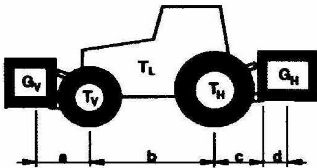
Abbildung 39: Schaubild Gewichtsverteilung
