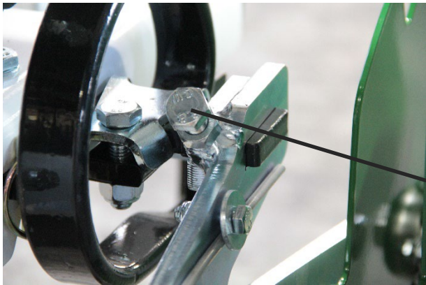
Abbildung 28: Scheibenmontage
