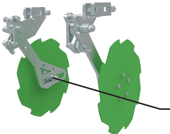
Abbildung 26: Scheibenlagerung
