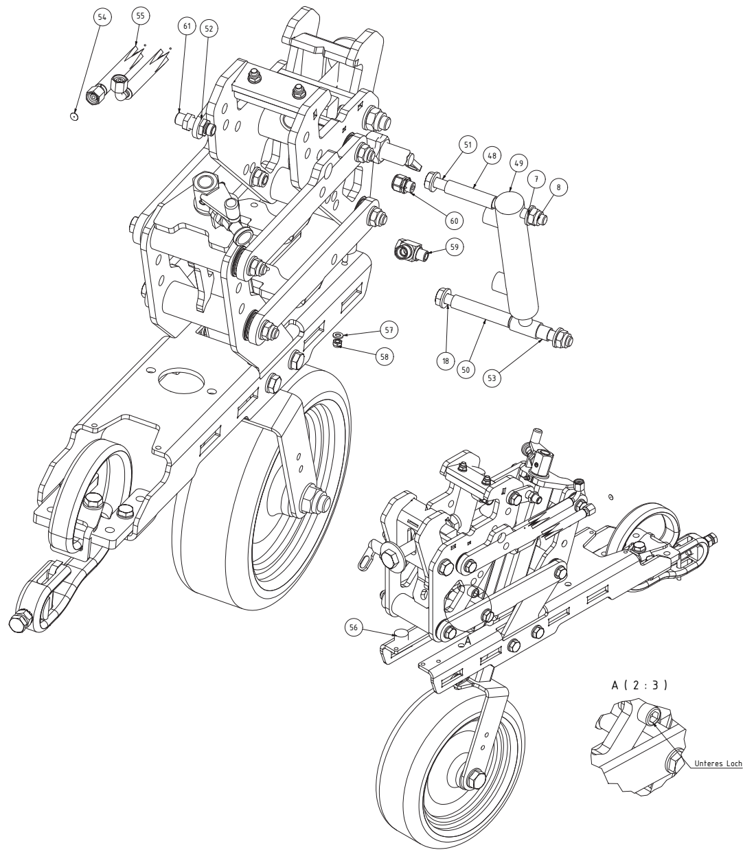
Montage Zinkenhackmodul laut Zeichnung 097608
